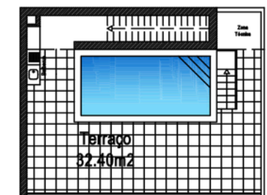
COBERTURA - ESQUERDO
