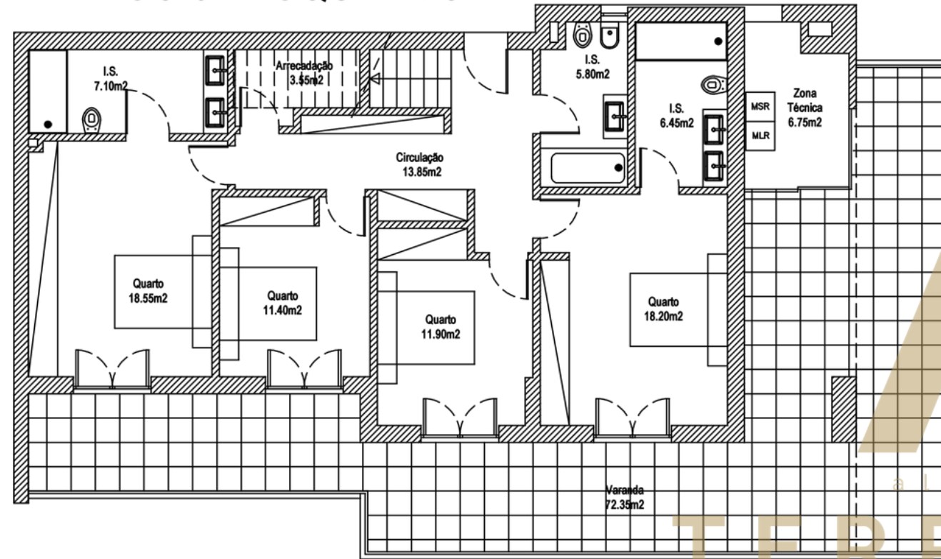
PISO 3 - ESQUERDO
